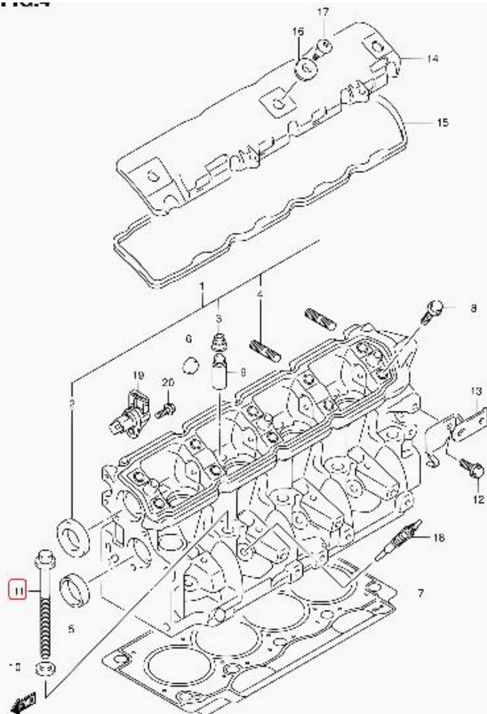
JB420W E22 004 CYLINDER HEAD (JB419)
