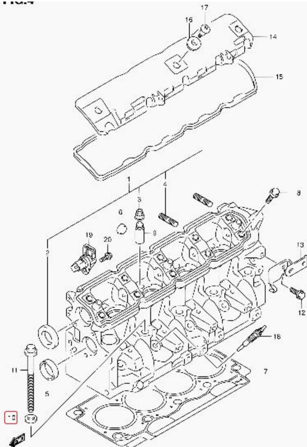
JB420W E22 004 CYLINDER HEAD (JB419)
