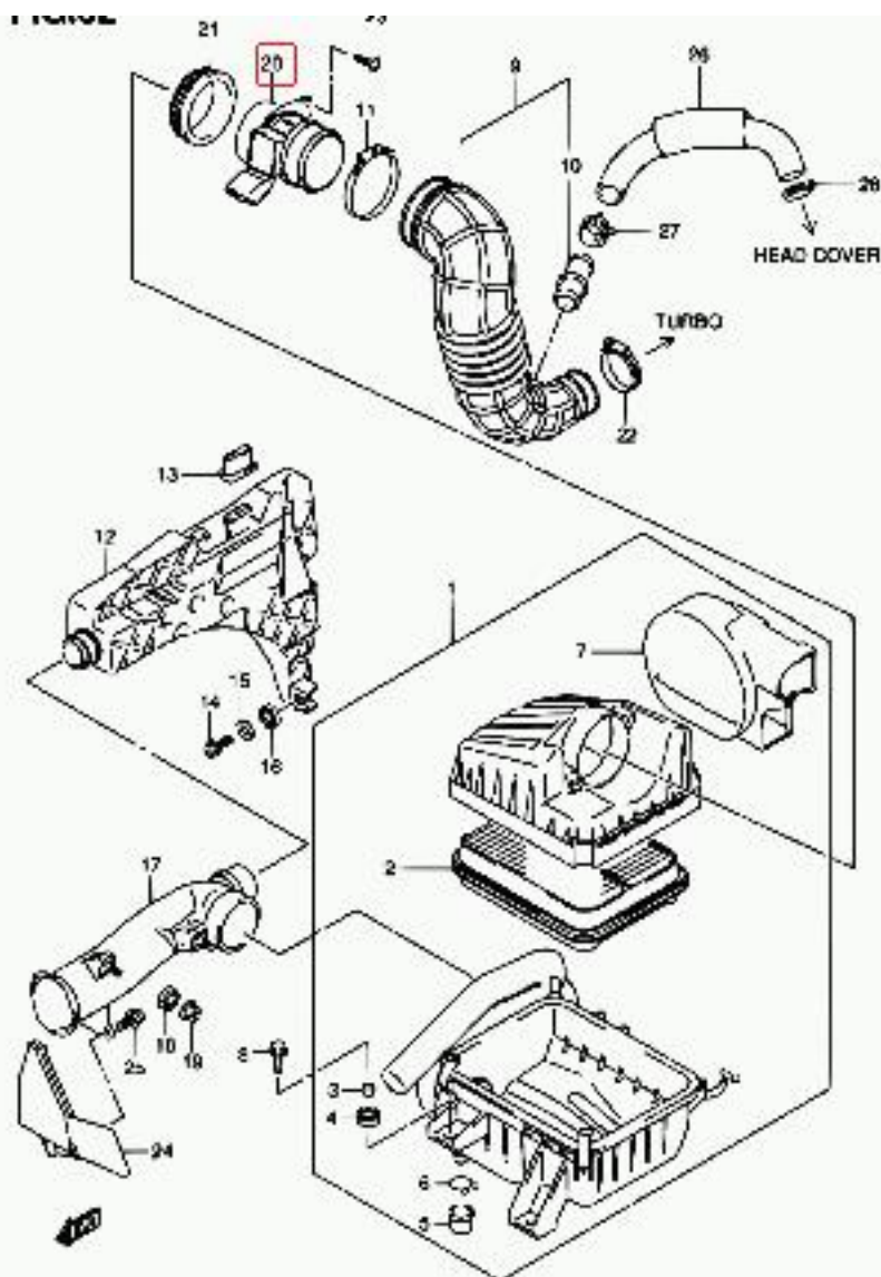
8Q420W-3 E22_c32 AIR CLEANER (8Q420WD)
