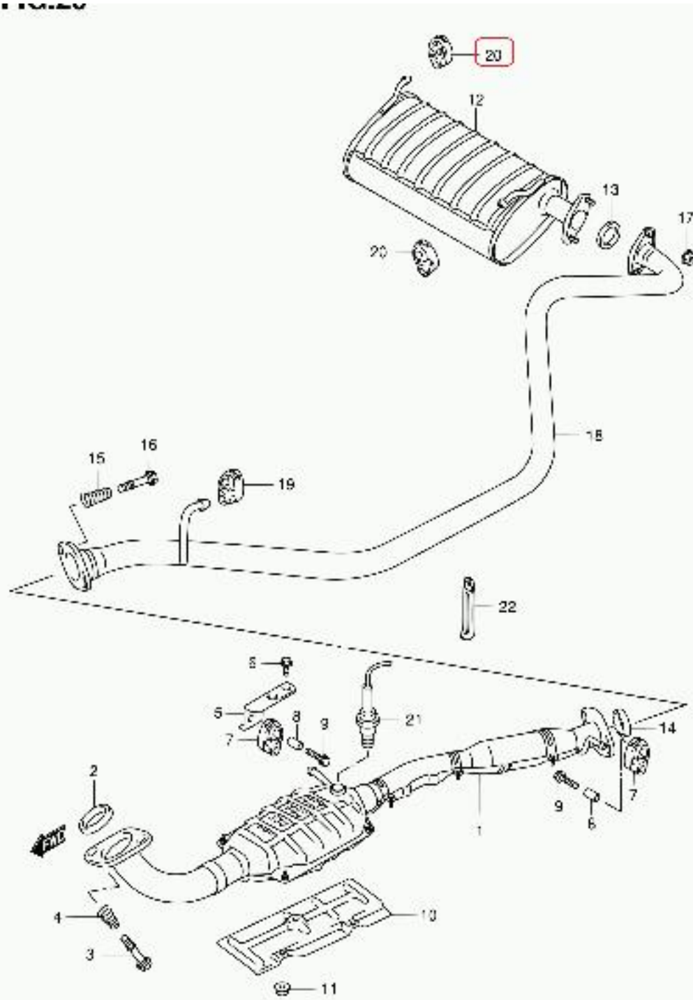
SK413V-2 E22 026 MUFFLER (SK413V)
