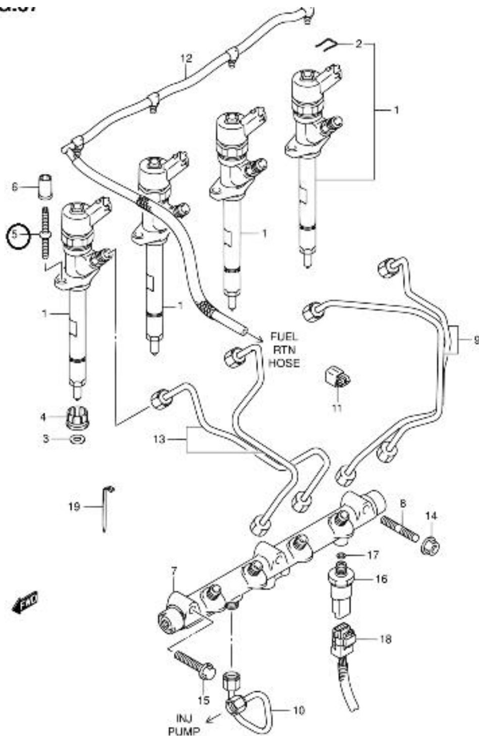
JA627W-4 E22 037 DELIVERY PIPE (JA420WD)
