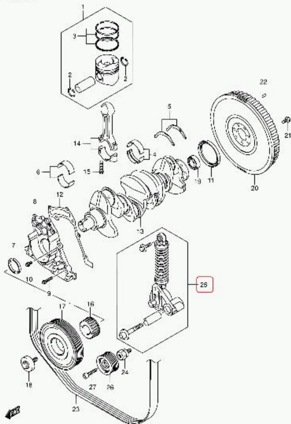
JB420W E22 012 CRANKSHAFT (JB418)
