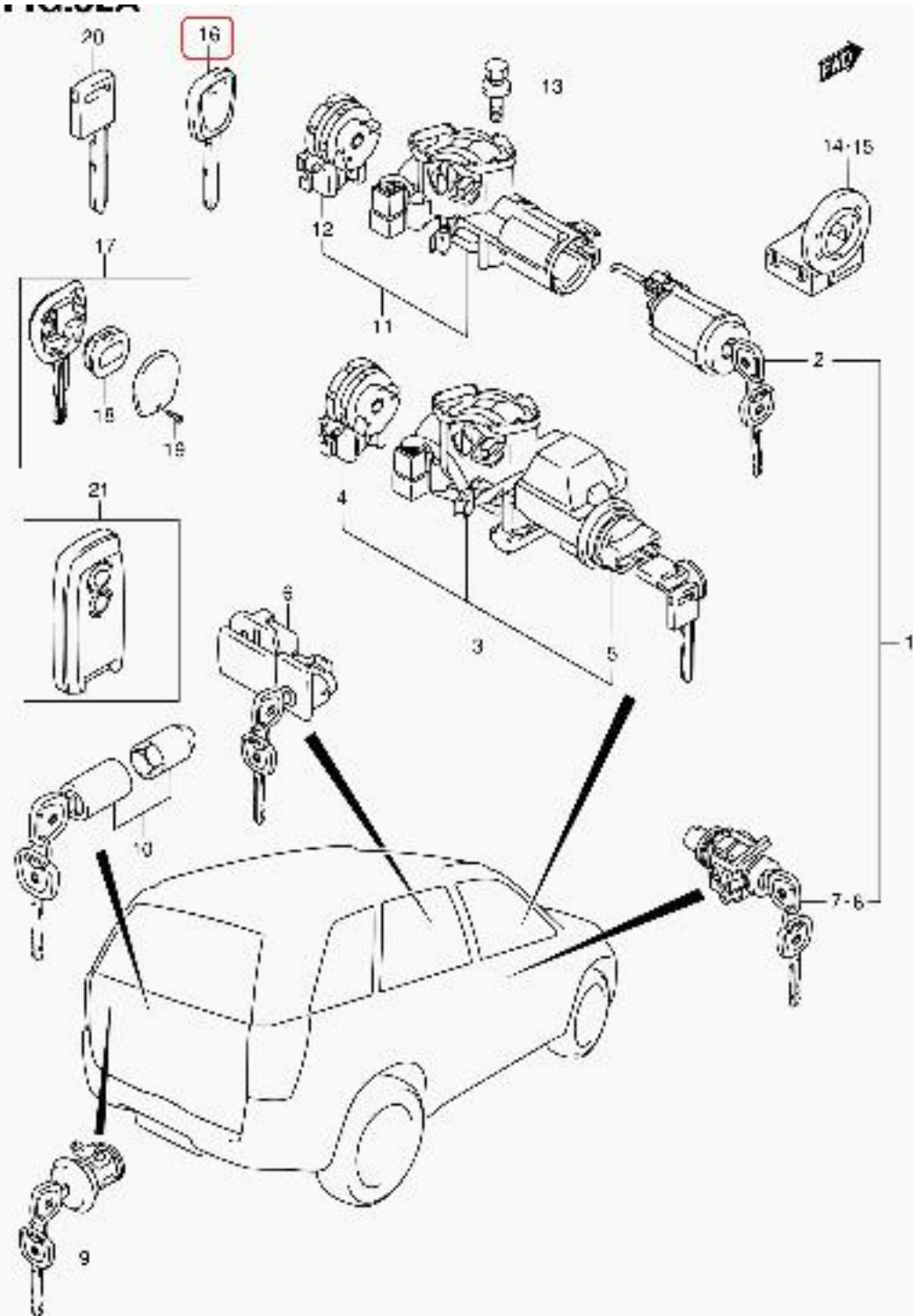
JB415X E22 082A LOCK SET (2)
