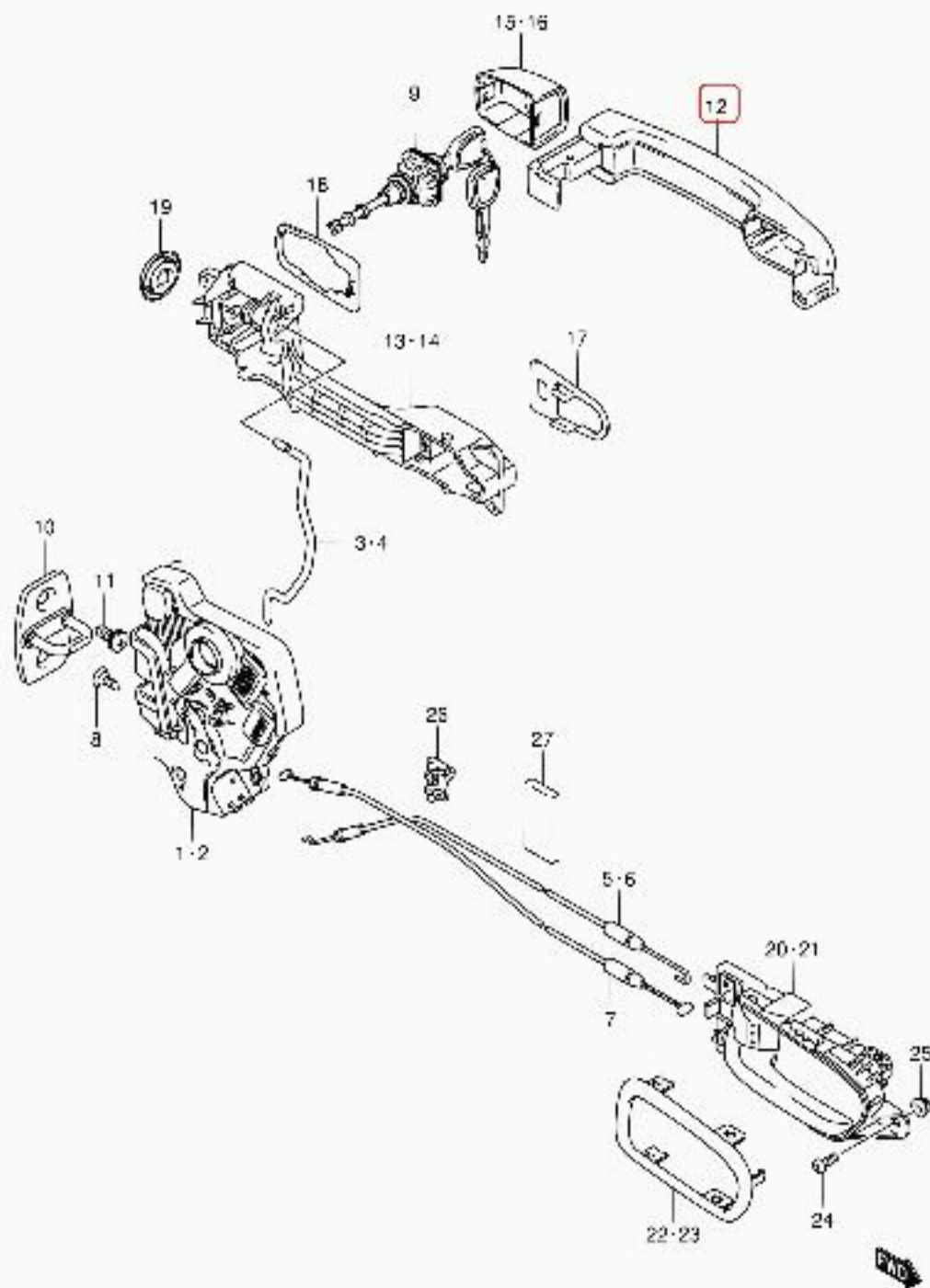
JB420W-4 E22 252 FRONT DOOR LOCK (1)
