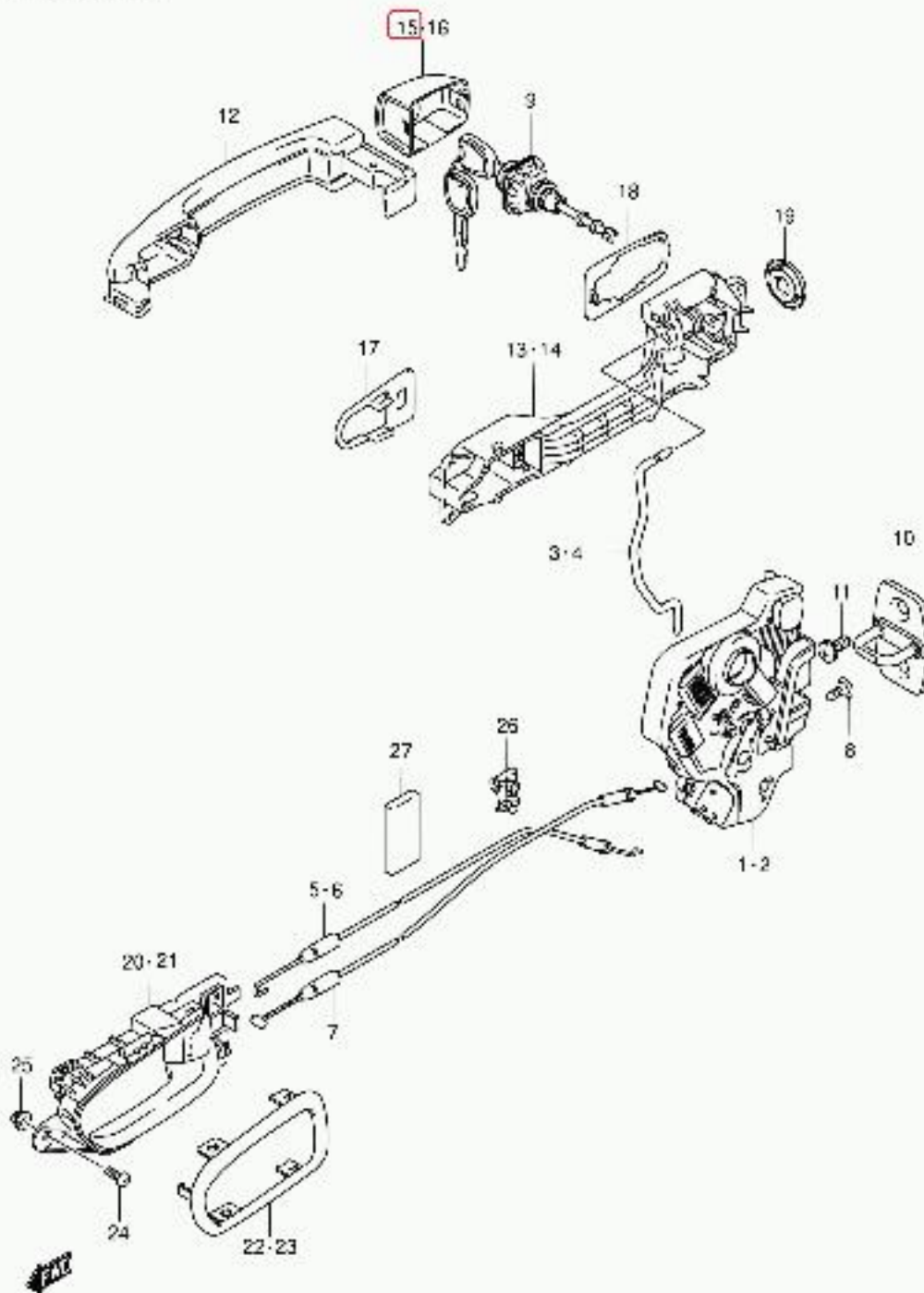
JS420W-4 E22 252A FRONT DOOR LOCK (2)
