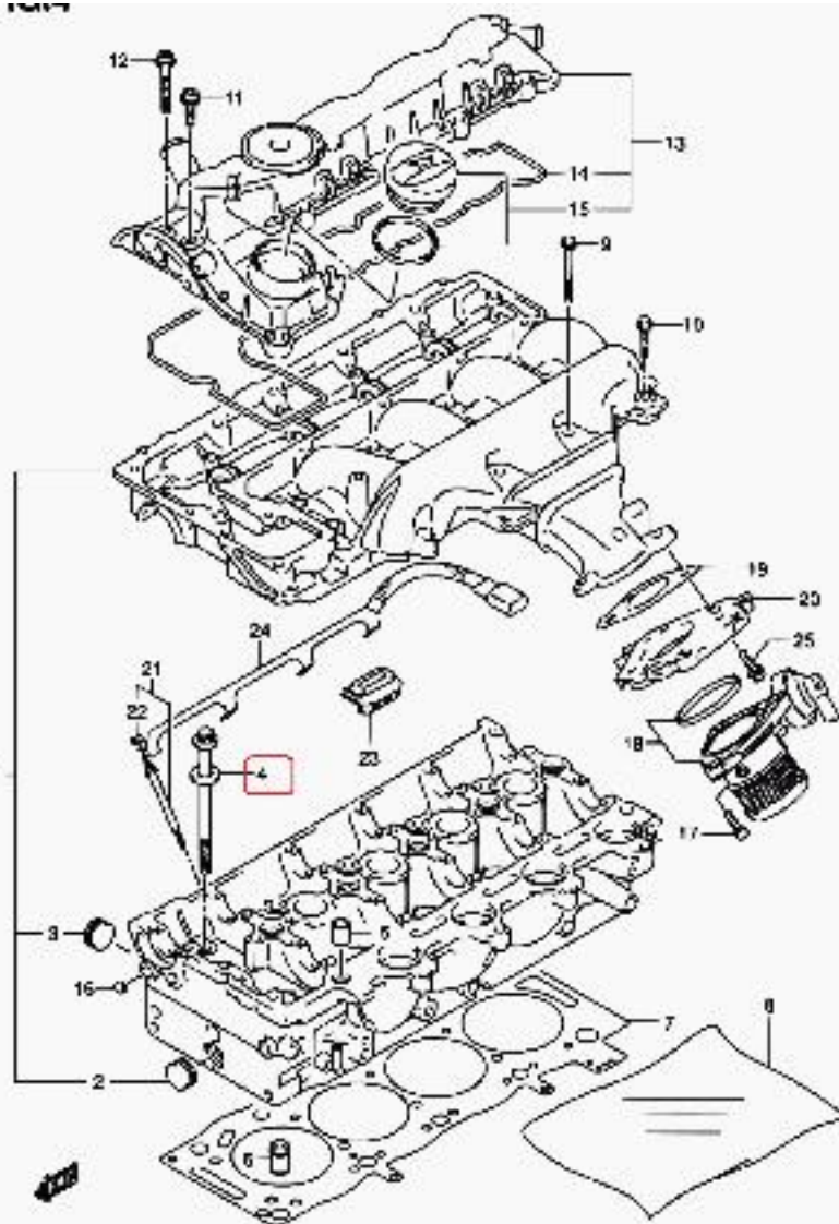
8Q420W-3 E22_504 CYLINDER HEAD (8Q420WD)
