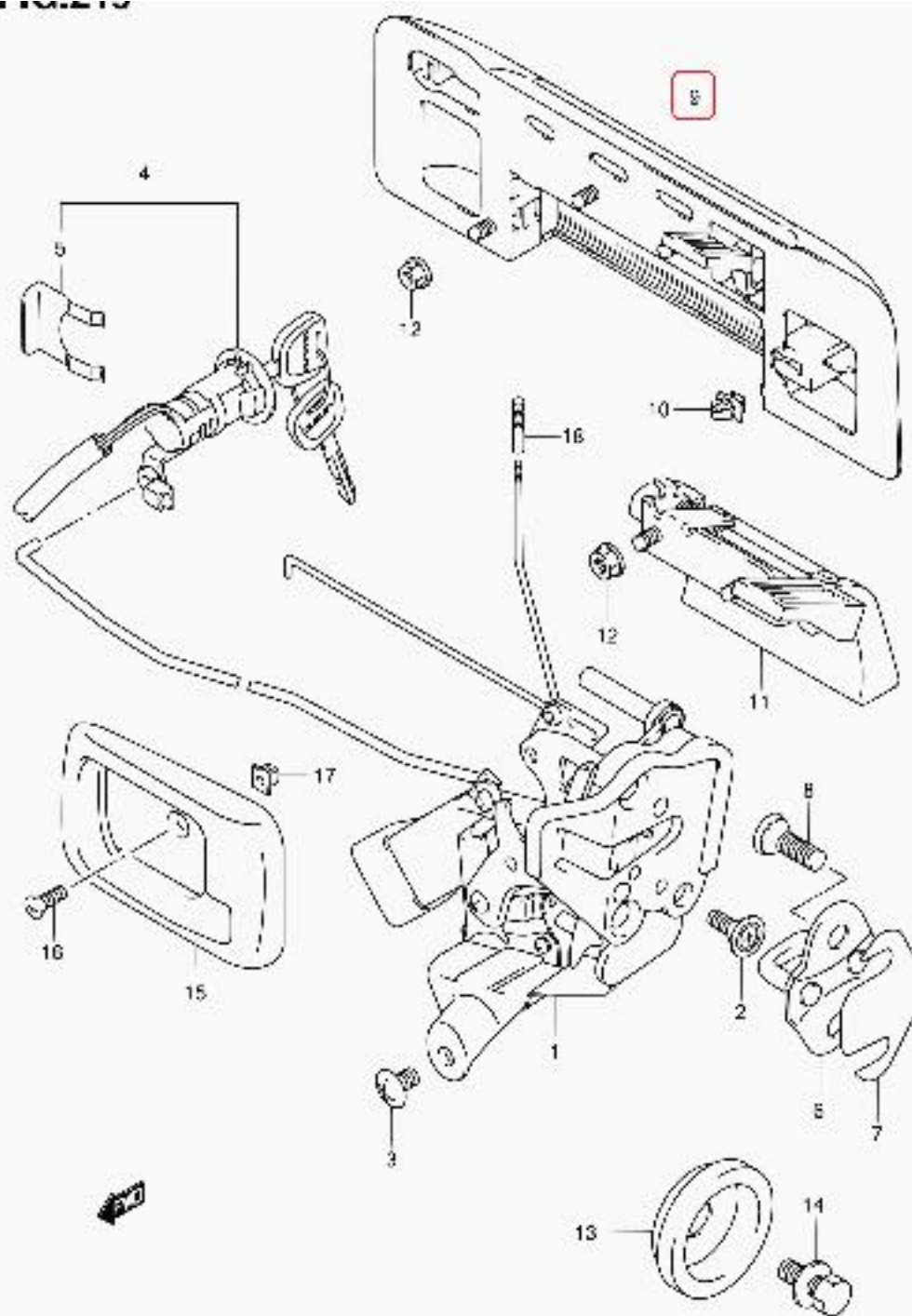
SQ416V-3 E22 219 BACK DOOR LOCK
