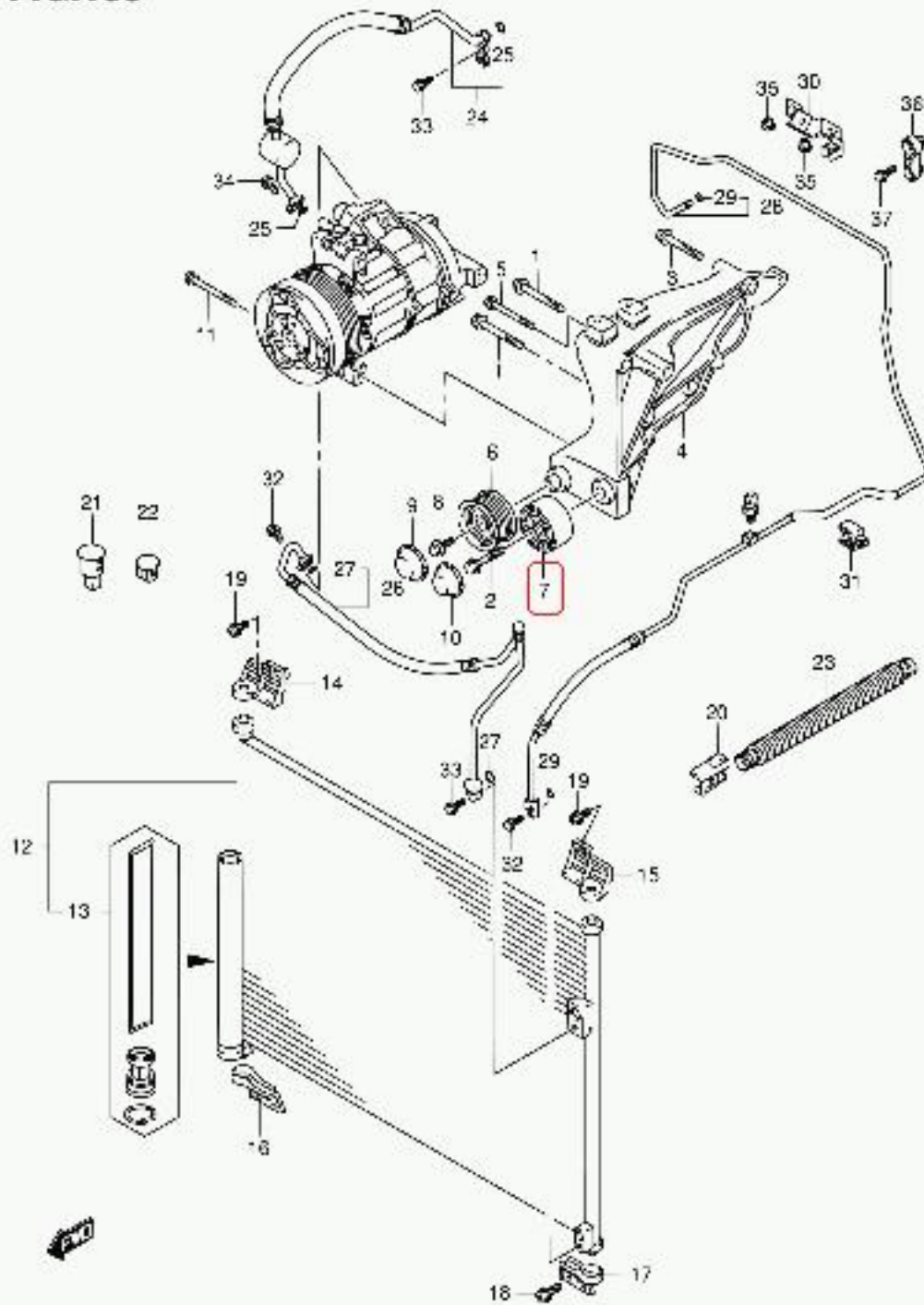
JB420W E22 163 AIR CON PIPING (2)
