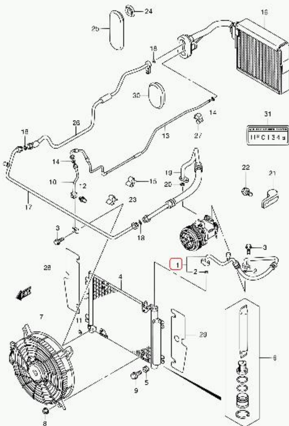
SQ416V-3 E22 230 AIR CON PIPING (1)
