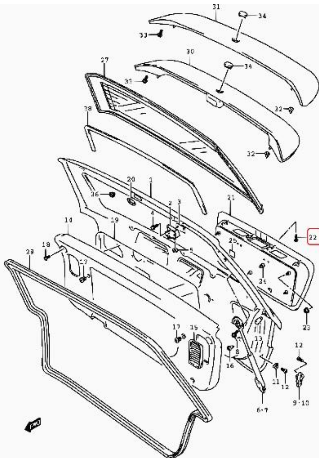
SY413-7 E01_296 5DR BACK DOOR PANEL
