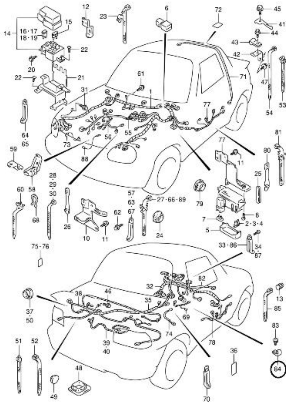
SZ416 E01 068 WIRING HARNESS (LHD)
