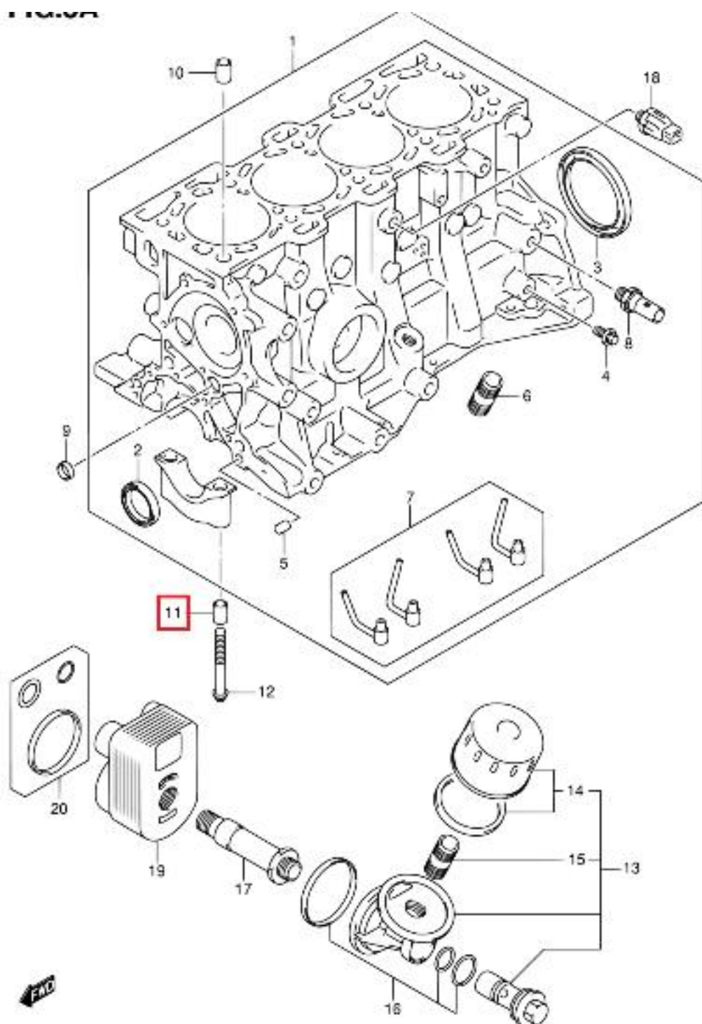
SN413V-5 E22 008A CYLINDER (3)
