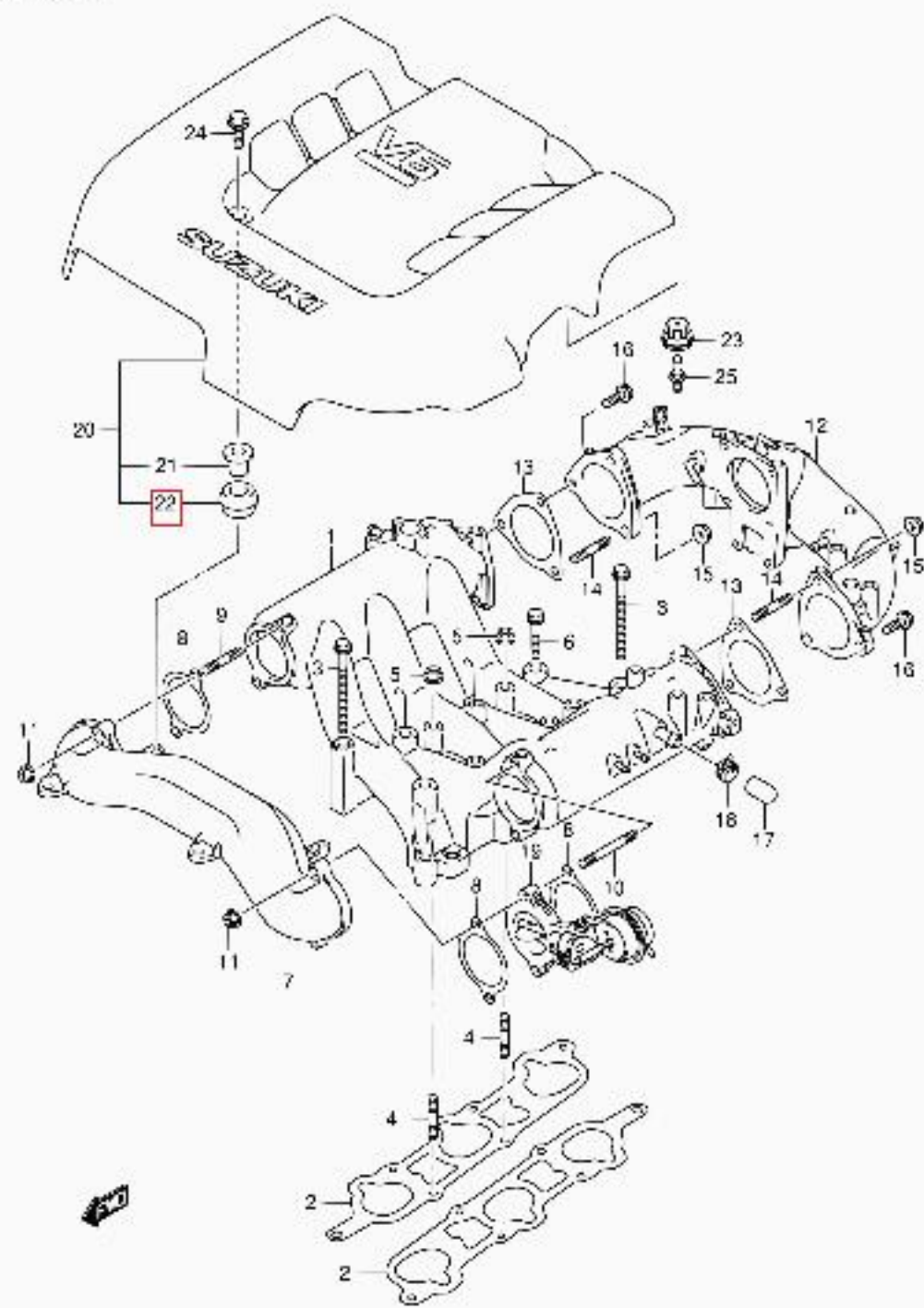
JB527W E26 009 INTAKE MANIFOLD
