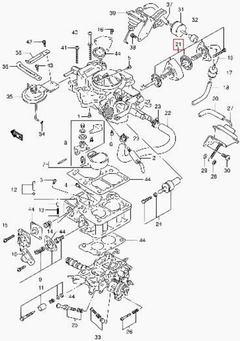
SE416 4 E01_026 CARBURETOR(MT E06,E21)
