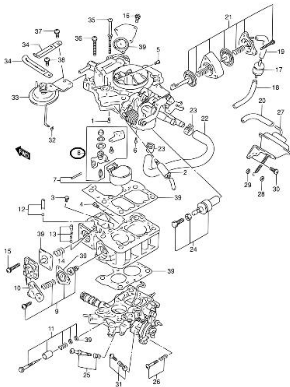
SE416 3DR E01 036 CARBURETOR (4)
