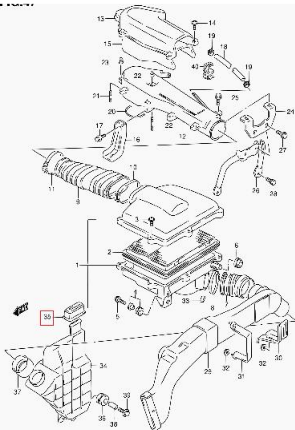
SE416 3DR E01 047 AIR CLEANER (4)
