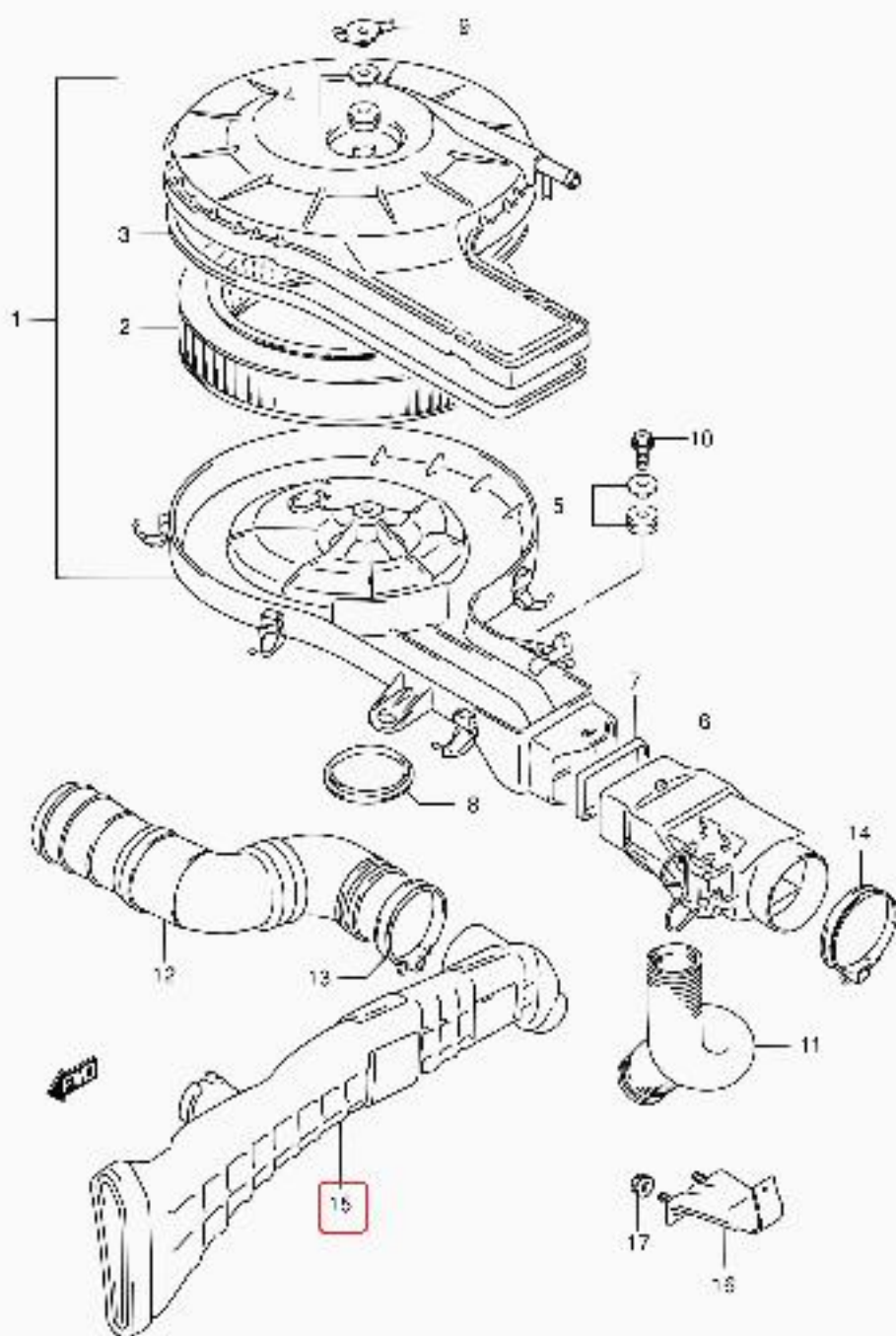
SE416 4 E01_032 AIR CLEANER(2V MT)
