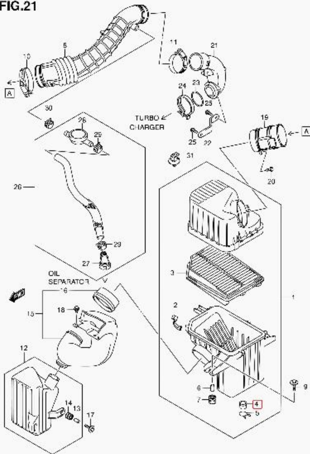
JB420W E22 021 AIR CLEANER (JB4119)
