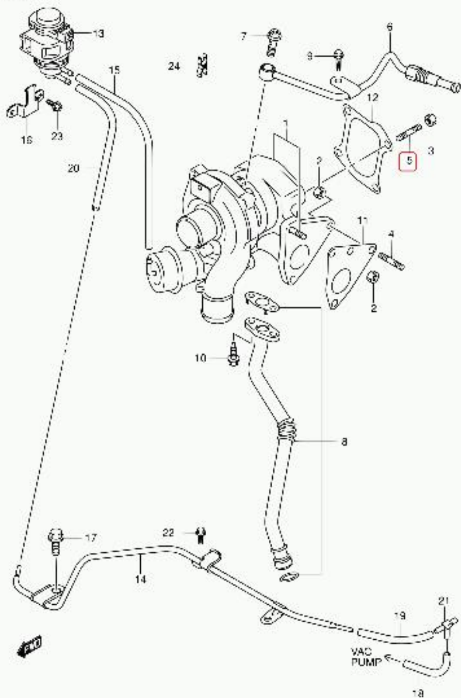
SN413V-5 E22 032A TURBO CHARGER (SN415VD:2)
