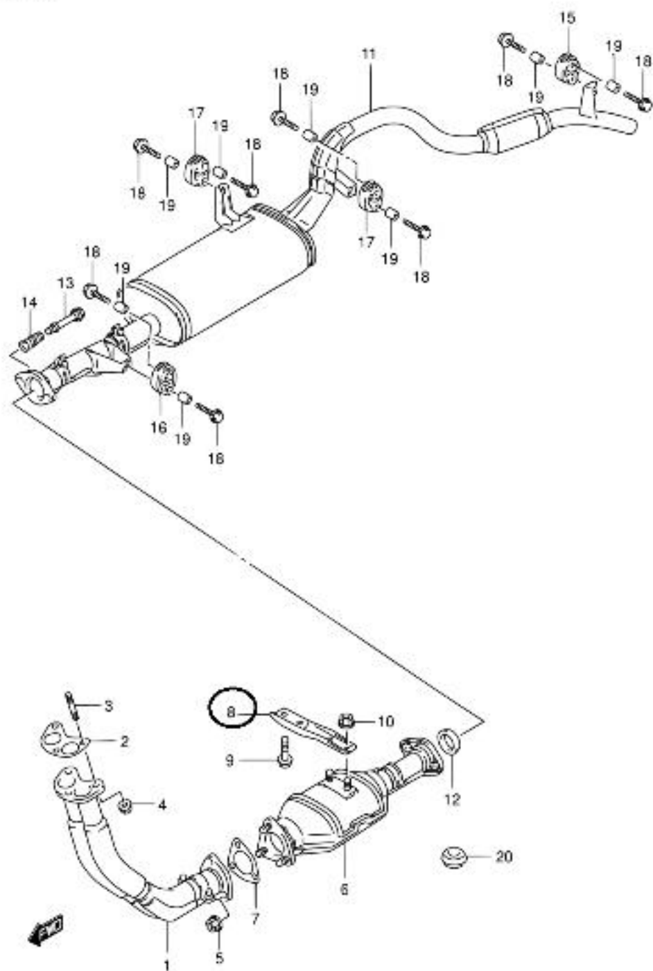
SE416-4 E01_040 MUFFLER(2V INJECTION)
