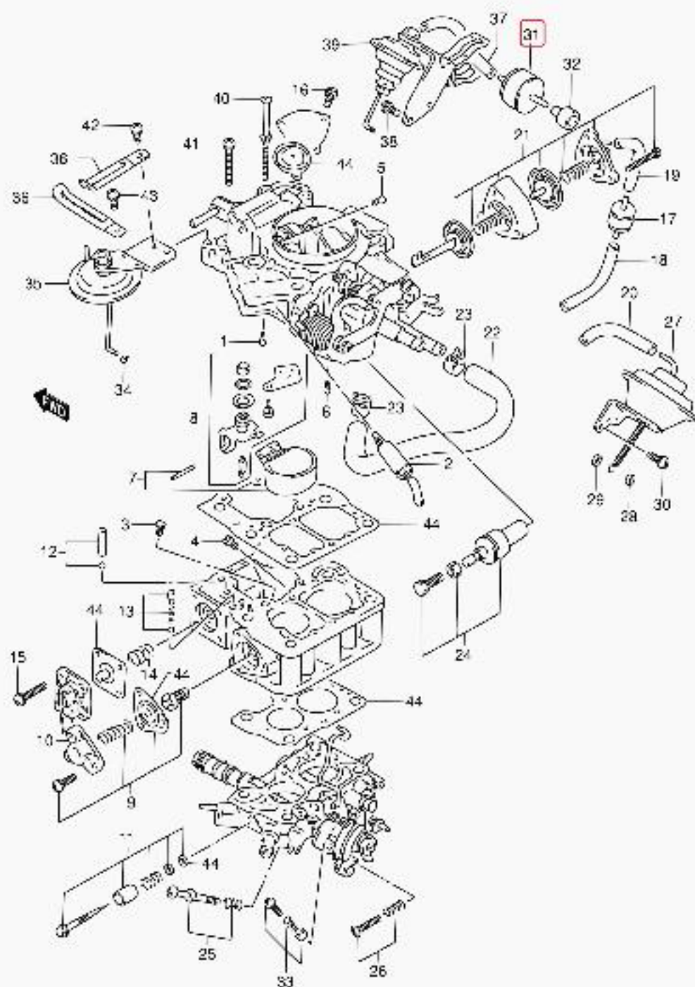
SE416 3DR E01 034 CARBURETOR (2)
