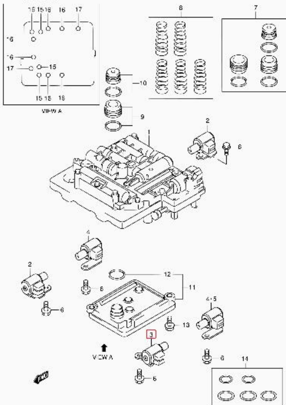
SN413V E22_033 VALVE BODY(AT)
