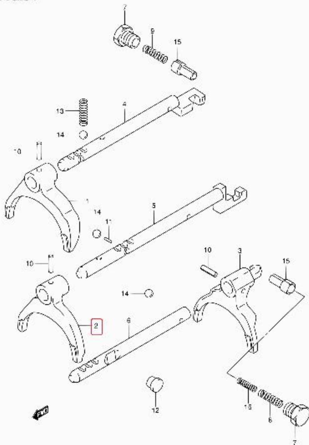
SN413V-2 E22 054 MT GEAR SHIFT FORK (MT SN413V)
