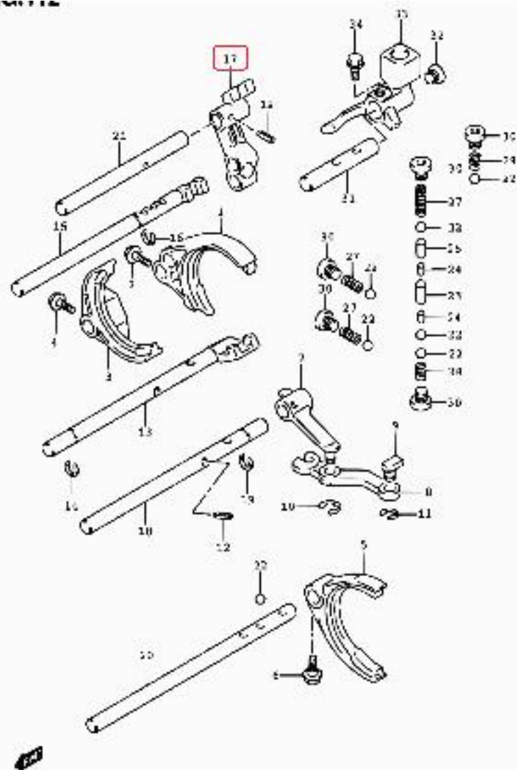
SG420M-2 E22_112 MT GEAR SHIFT FORK (MT:SG420MD;RT:SG42TM)
