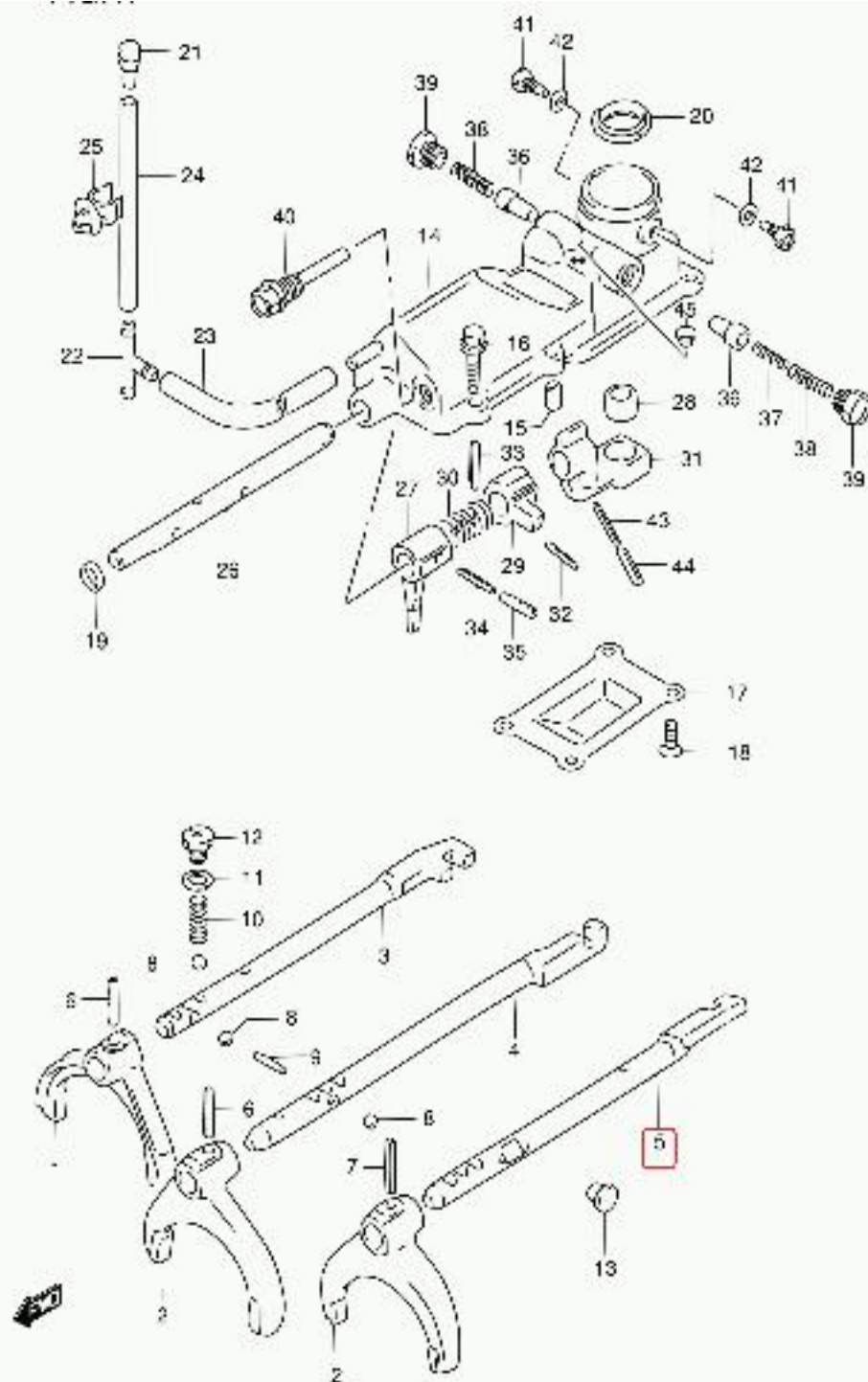
SO4200 E22_047 MT GEAR SHIFT FORK(MT)
