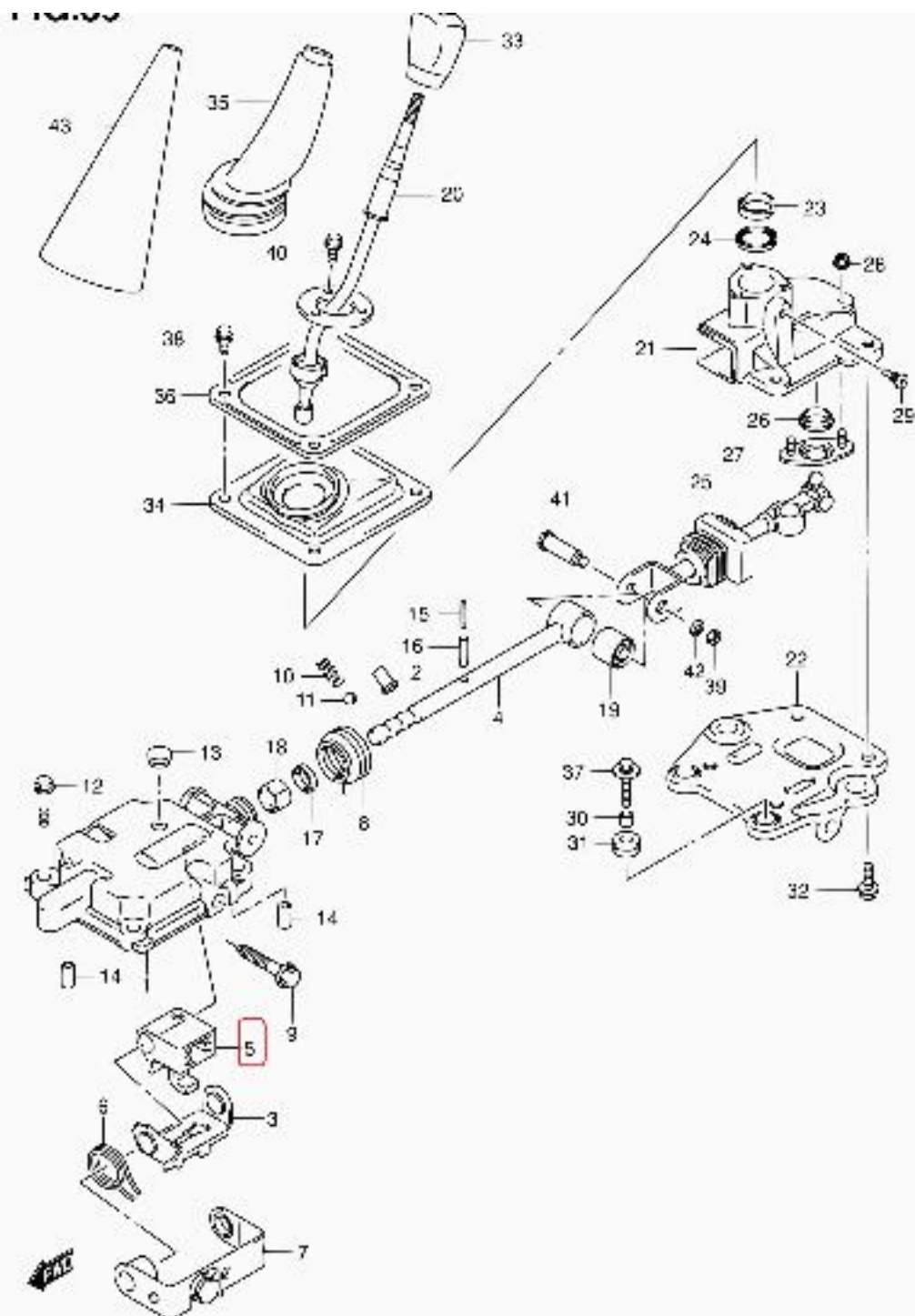
JB527W E26 039 GEAR SHIFT CONTROL (M T )
