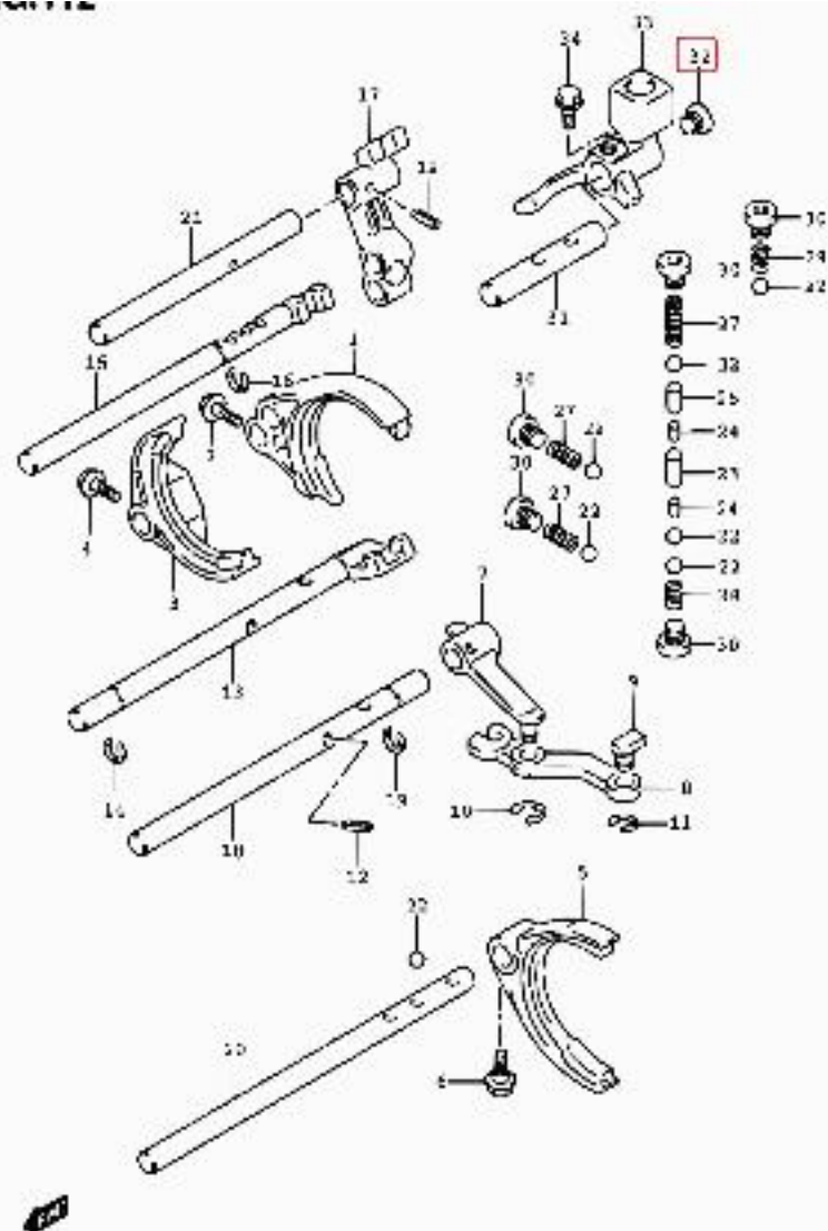
SG420M-2 E22_112 MT GEAR SHIFT FORK (MT:SG420MD;RT:SG421M)
