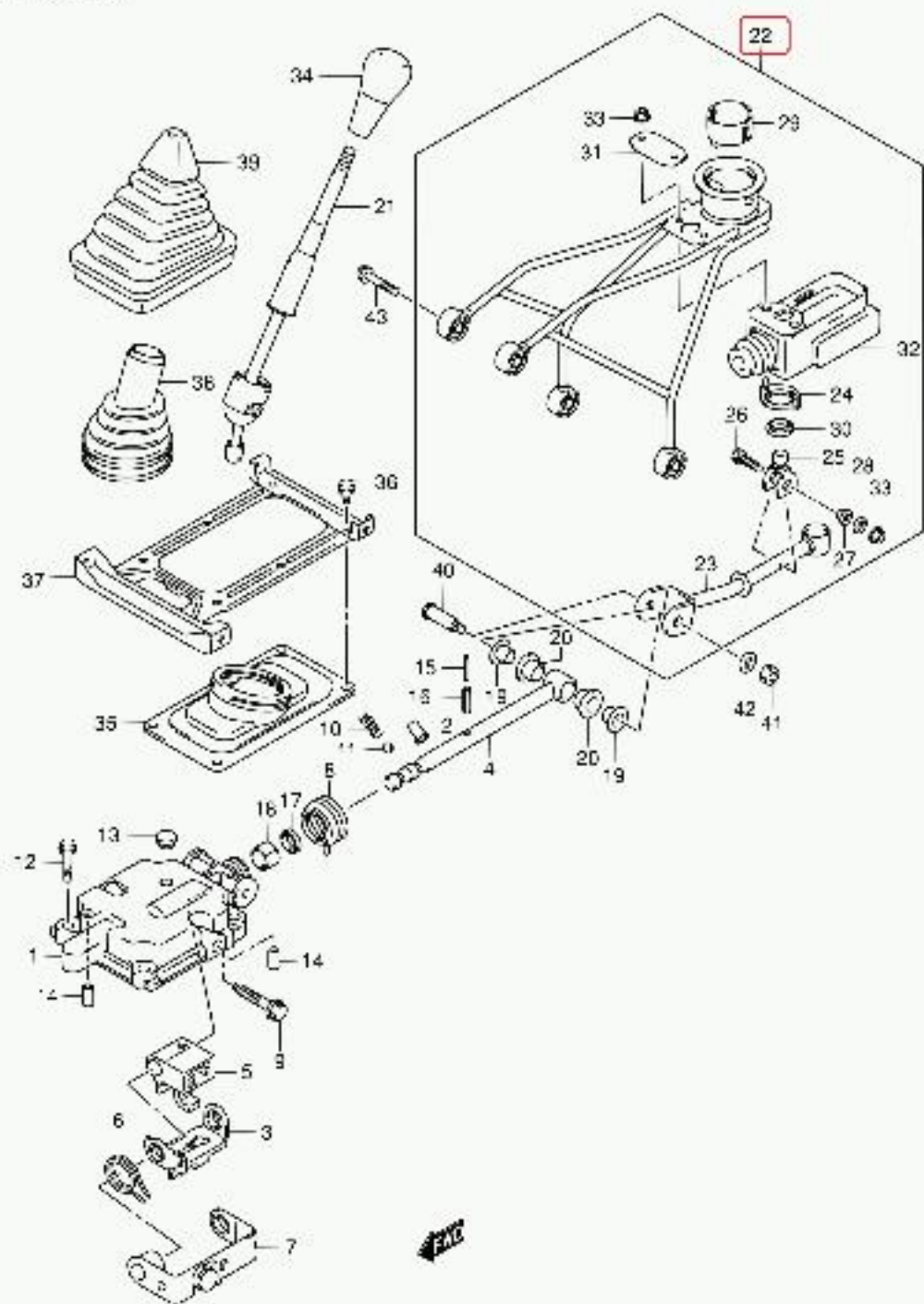
SA413V-5 E22 073 GEAR SHIFT CONTROL(2)
