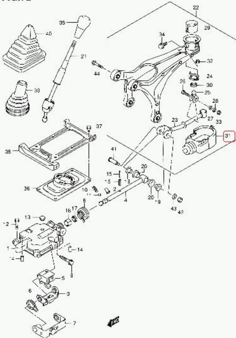
SA413V-5 E22 072 GEAR SHIFT CONTROL (1)
