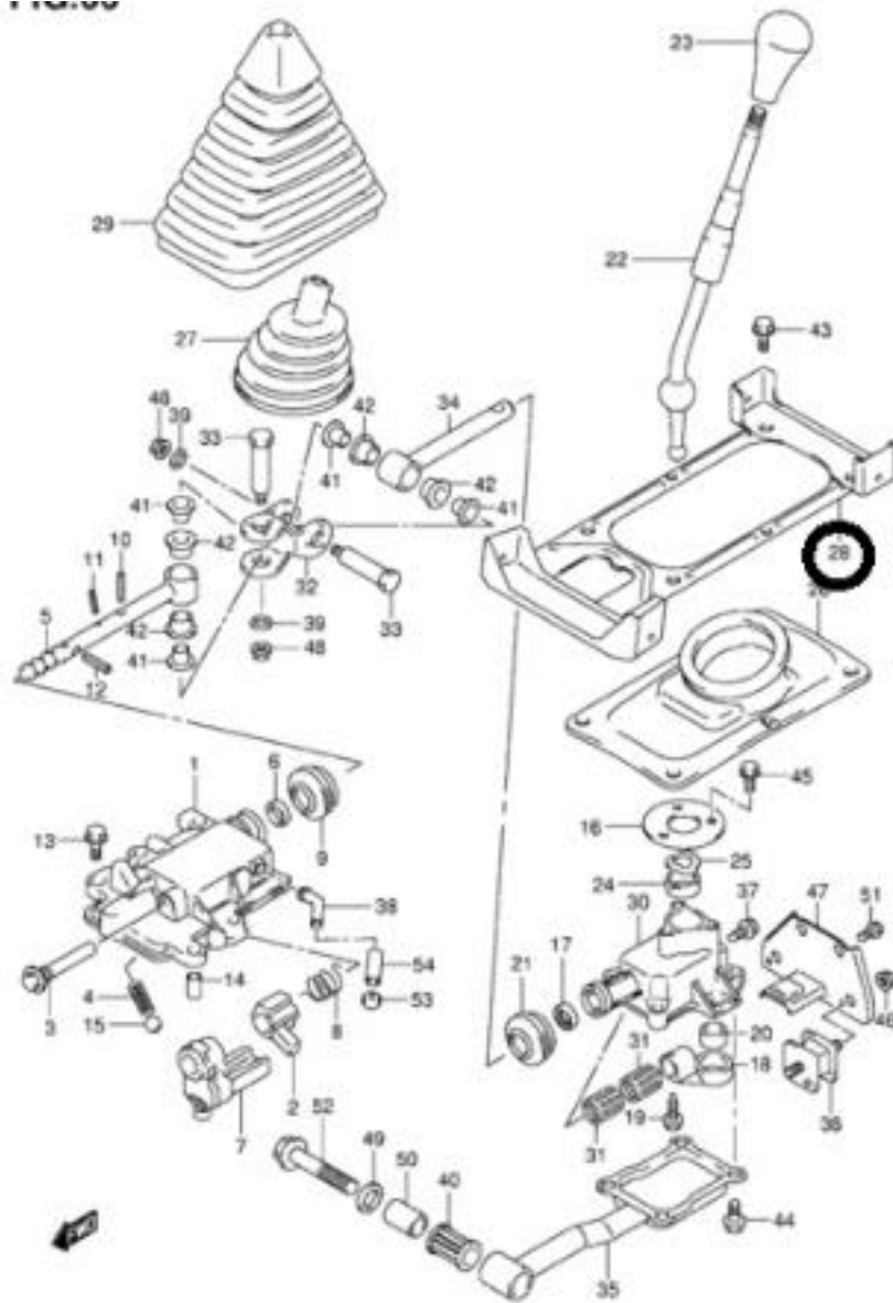
SN413V-2 E22_066 GEAR SHIFT CONTROL (MT:SN413V)
