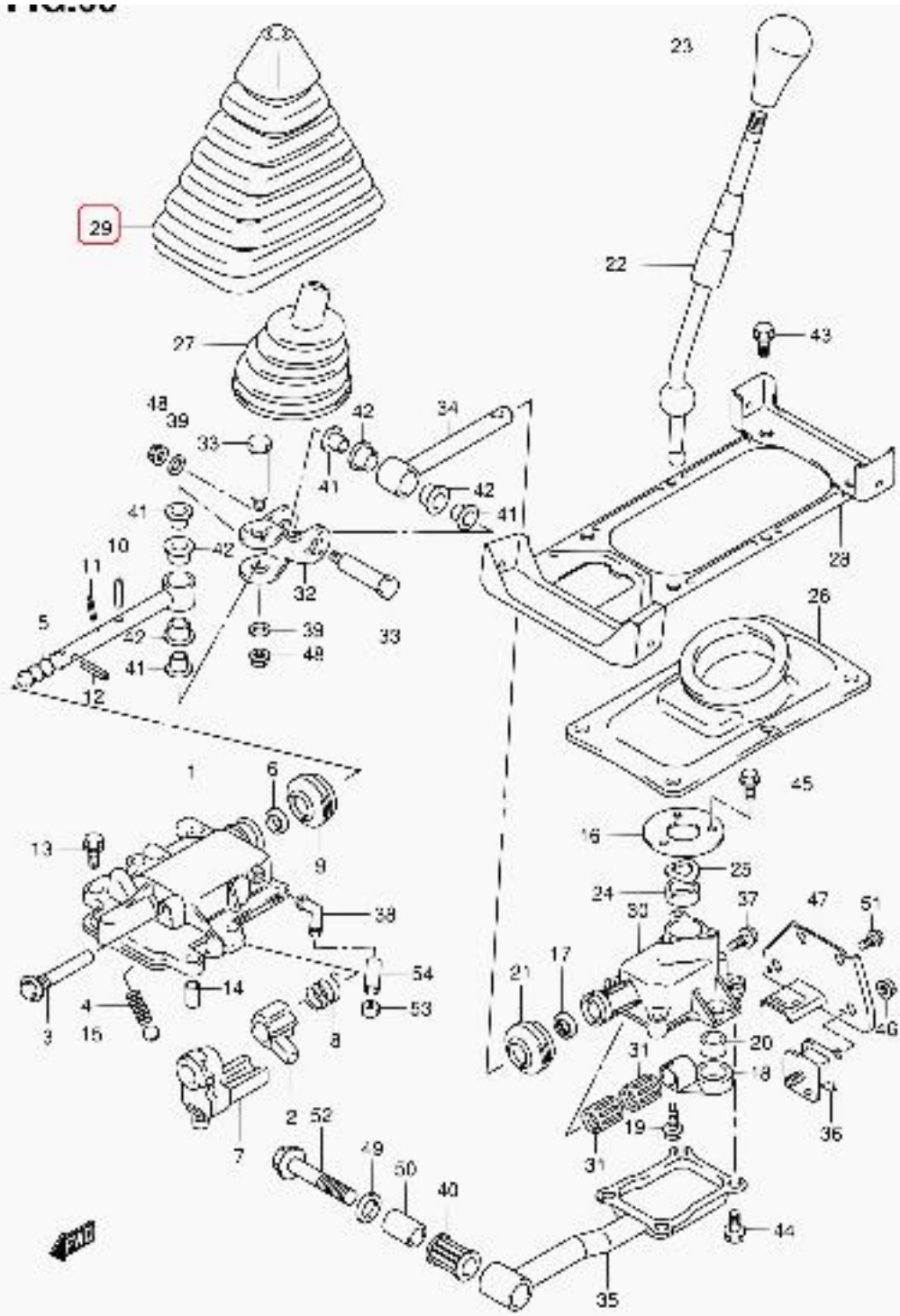
SN413V-2 E22 066 GEAR SHIFT CONTROL (VT SN413V)
