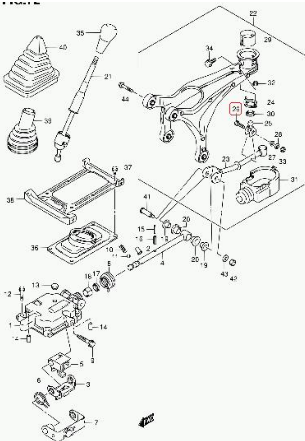
SK413V-5 E22 072 GEAR SHIFT CONTROL(1)
