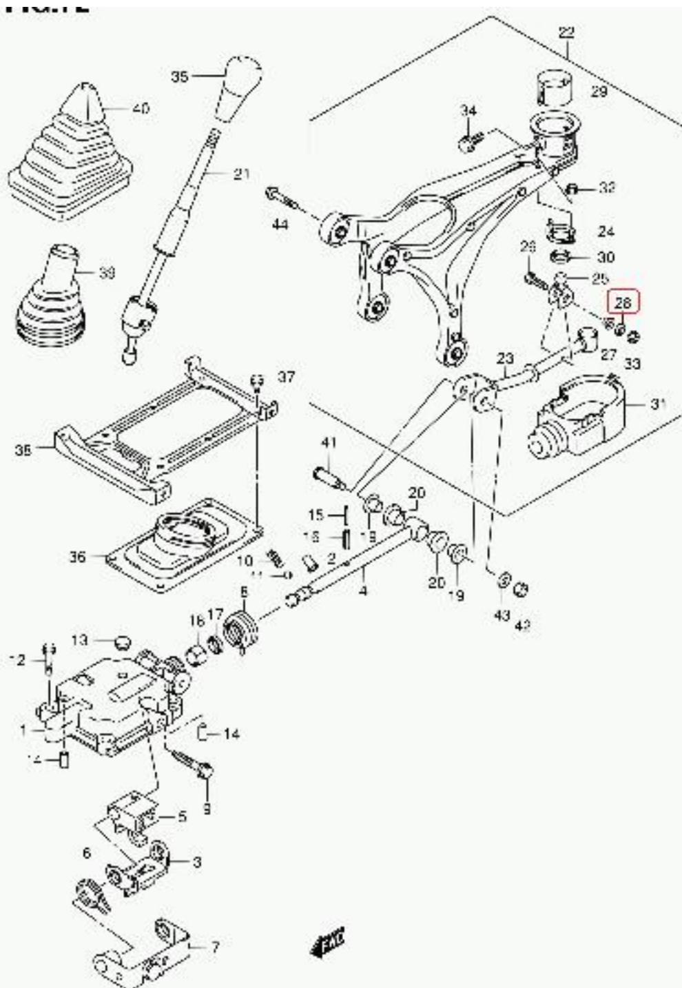
SK413V-6 E22 072 GEAR SHIFT CONTROL (1)
