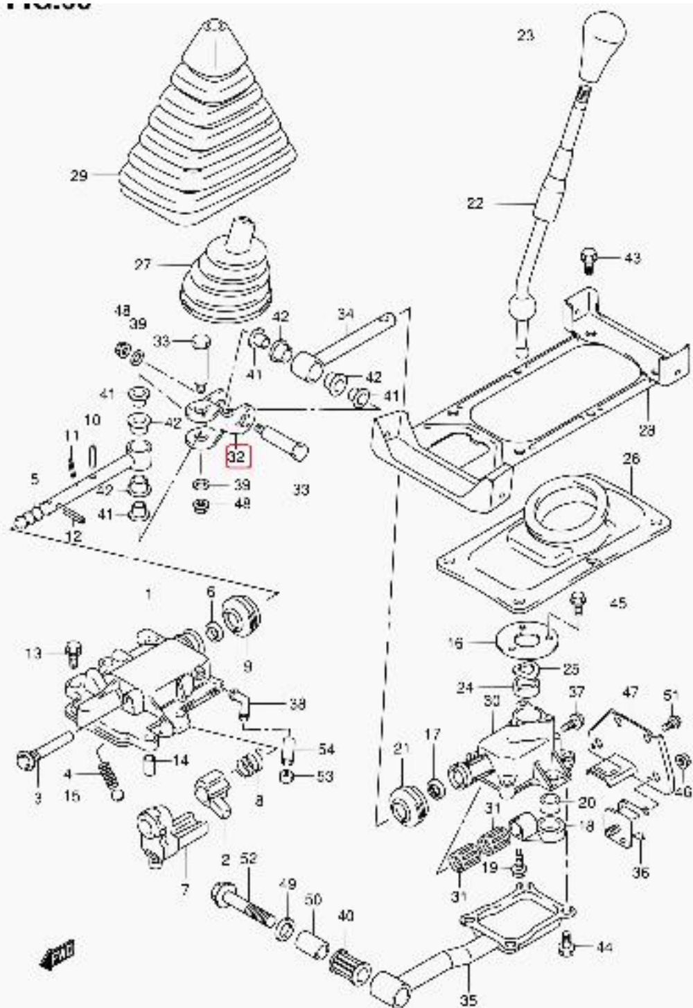
SN413V-2 E22 065 GEAR SHIFT CONTROL (VT-SN413V)
