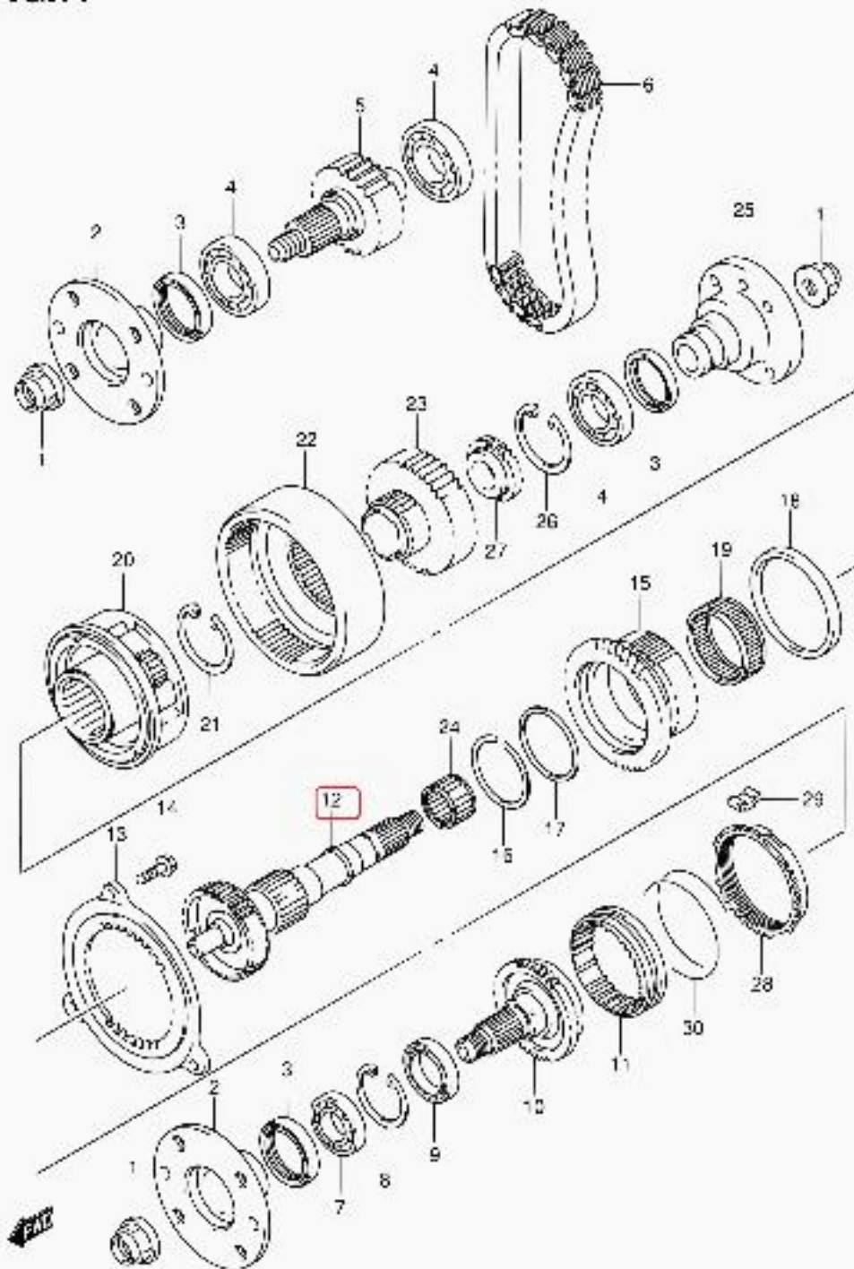
SN413V-2 E22 077 TRANSFER GEAR (4WD:SN413V)
