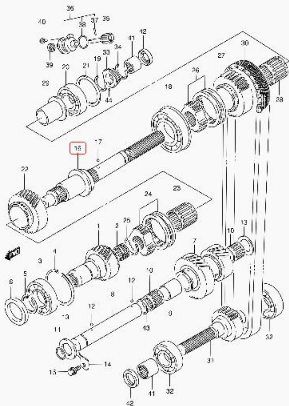
SE416 4 E01_103 TRANSFER GEAR
