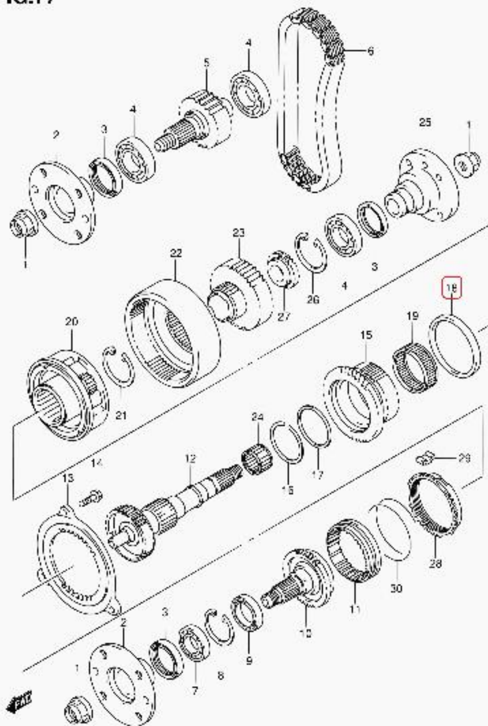
SK413V-2 E22 077 TRANSFER GEAR (4WD:SK413V)
