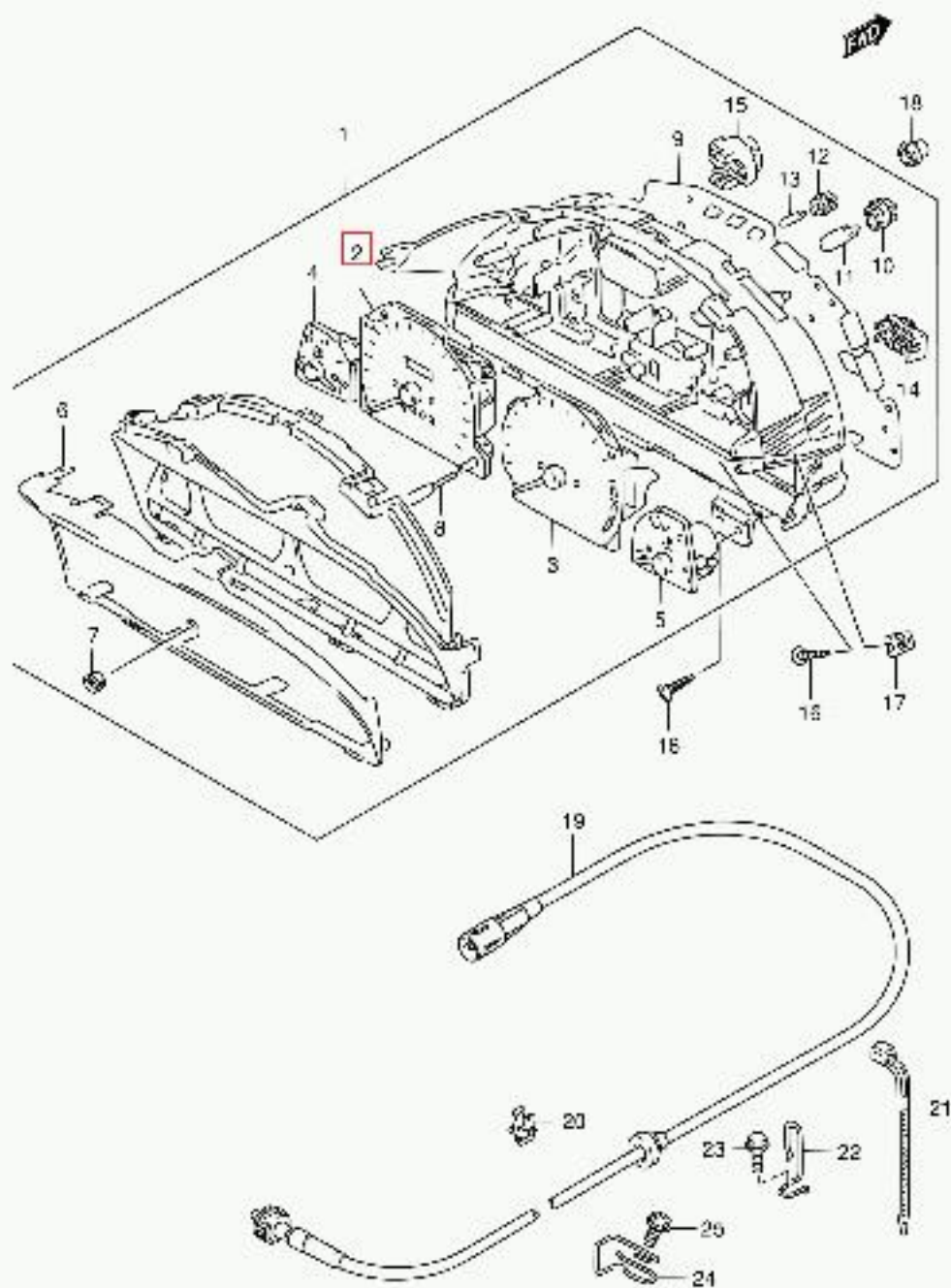
SE416 4 E01_115 SPEEDOMETER
