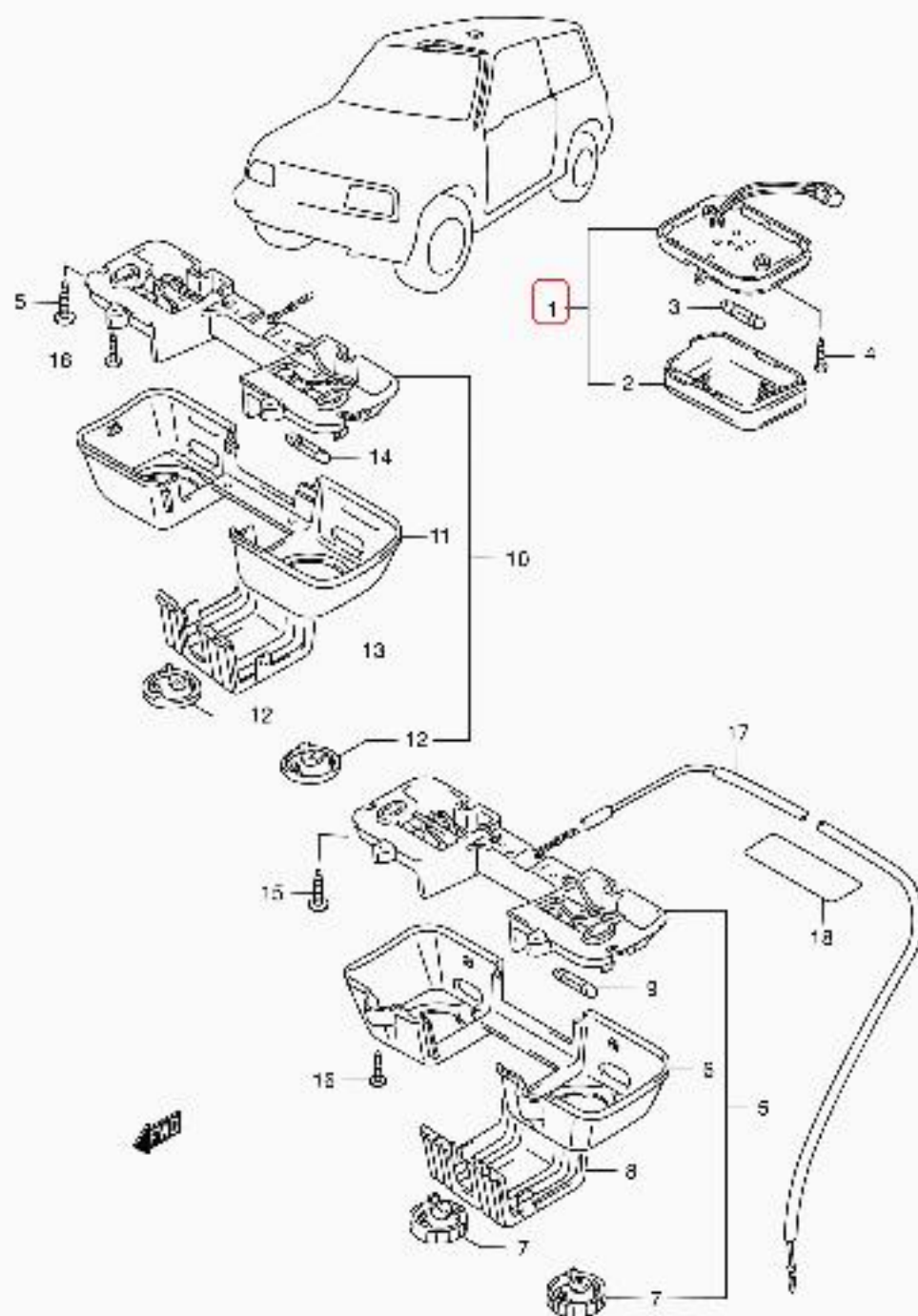
SE416 4 E01_117 ROOM LAMP
