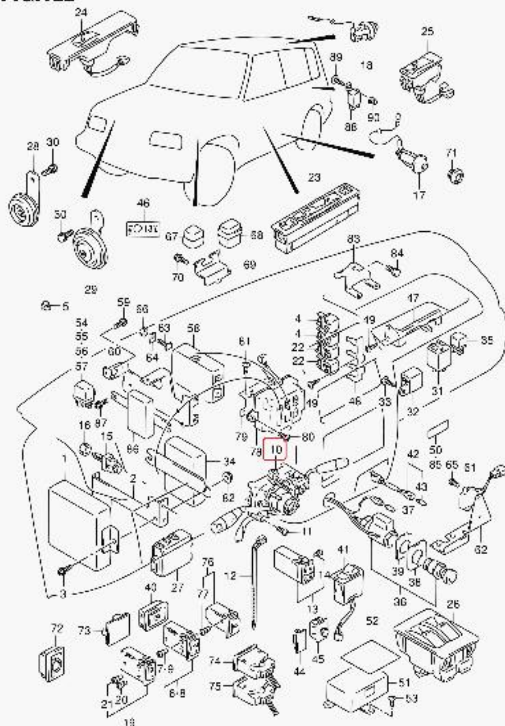
SE416 4 E01_122 ELECTRICAL CONTROL (LHD)
