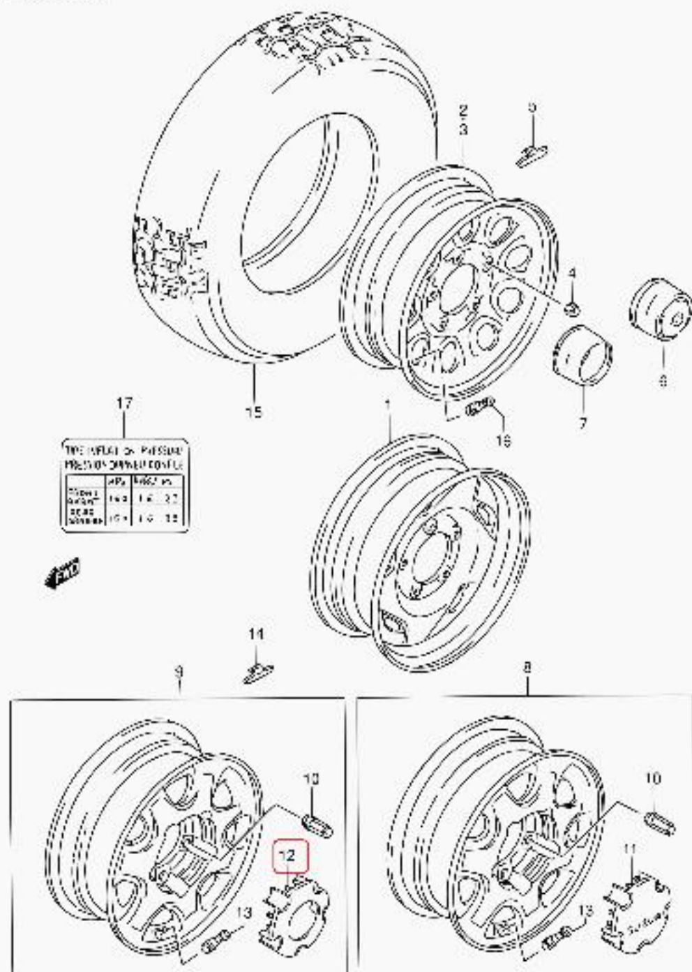
SE416 3DR E01 183 ROAD WHEEL
