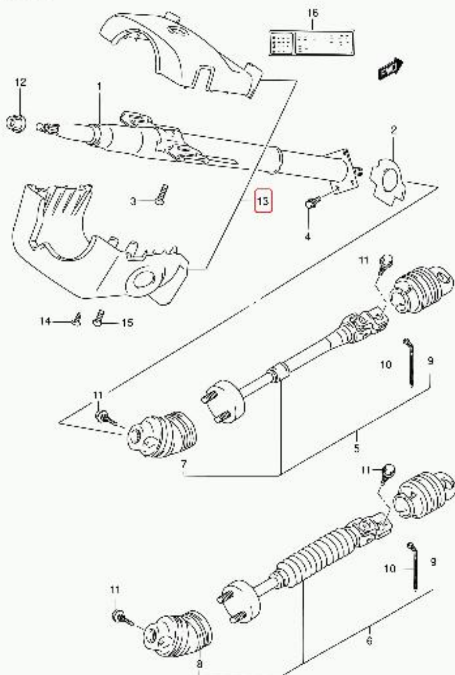
SE416 4 E01_141 STEERING COLUMN
