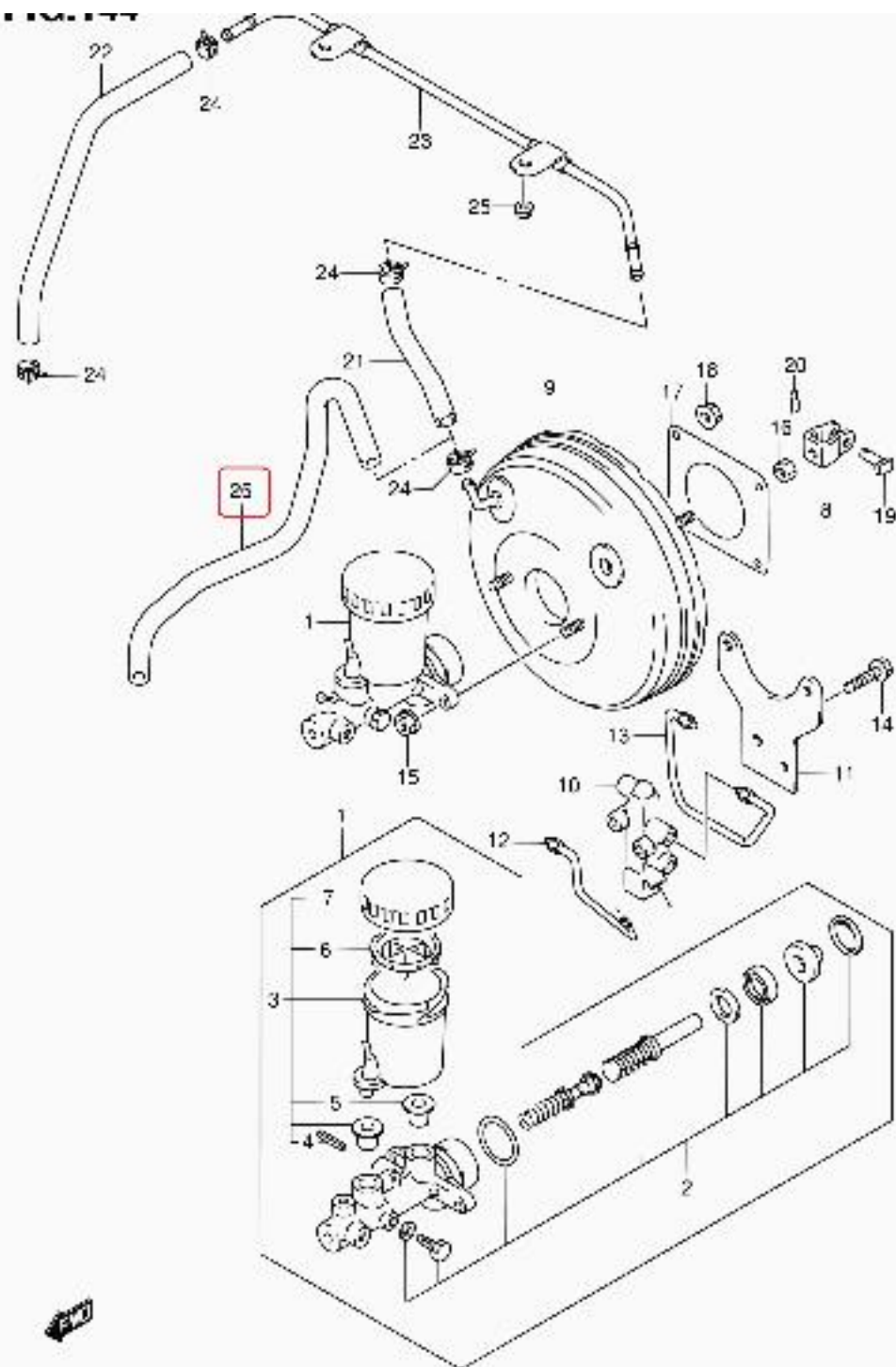
SA413V-2 E22 144 BRAKE MASTER CYLINDER (LHD)
