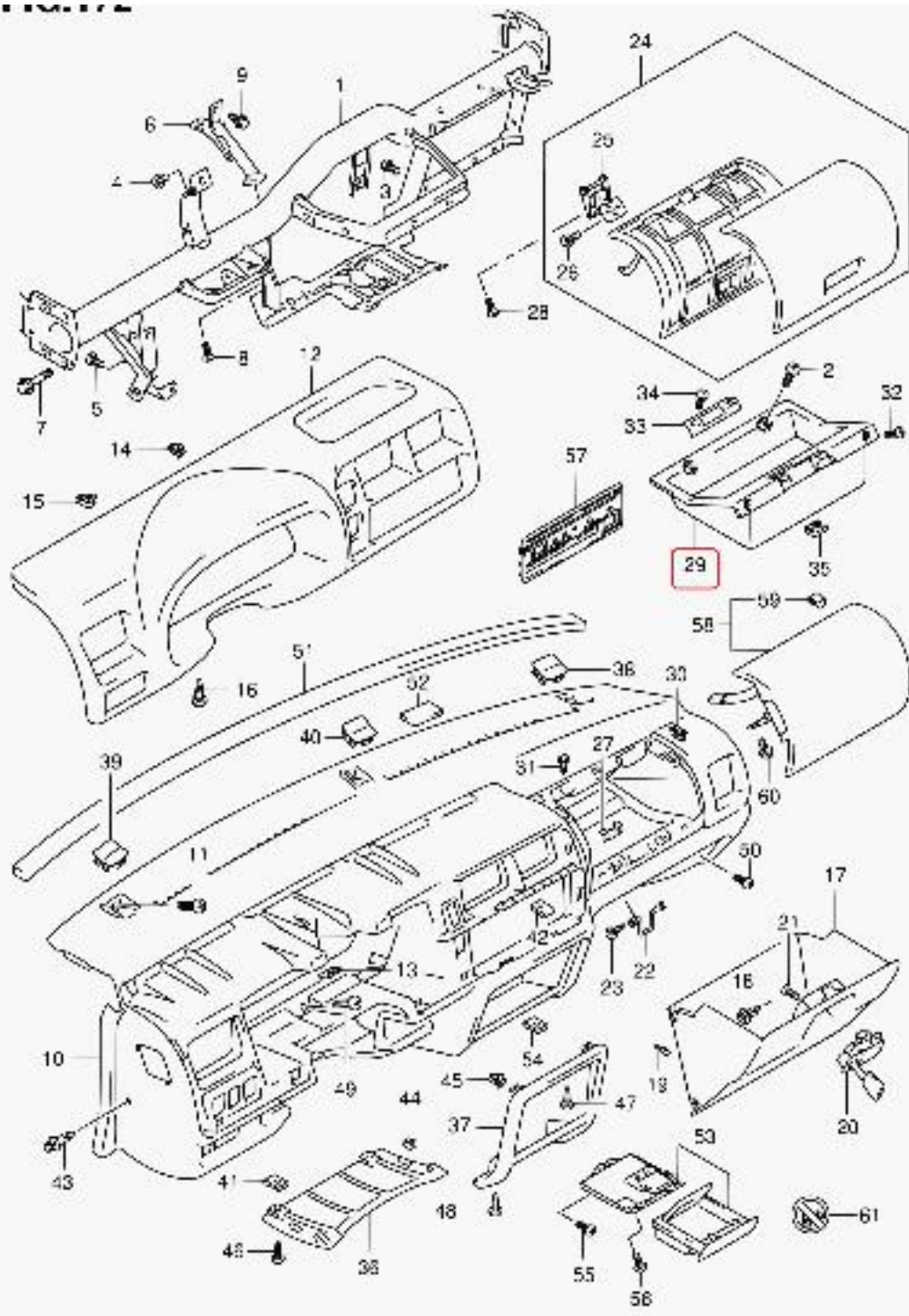
SN413V-2 E22 172 INSTRUMENT PANEL (.HD)
