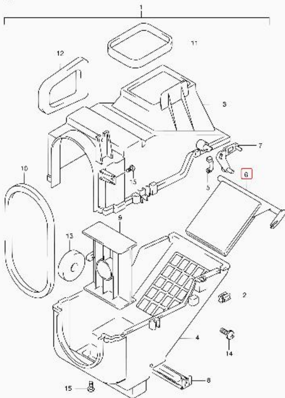
SN413V-2 E22 178 AIR INLET BOX (LHD)
