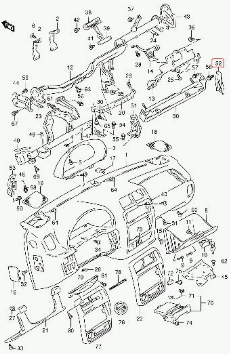
SE416 4 E01_189 INSTRUMENT PANEL (LHD: AIR BAG)
